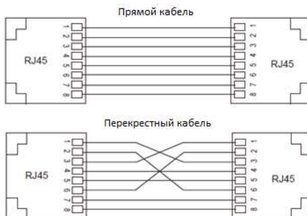
Рис. 7. Схема кабелей
